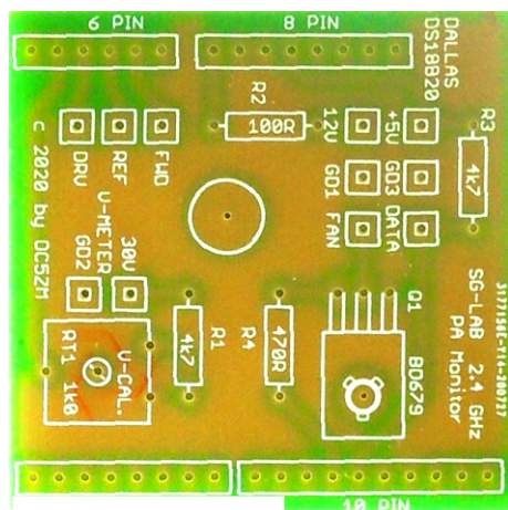
UNO PCB
